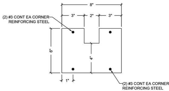
6 END COLUMN SECTION 6x8 SCALE: 3"=1'-0"
