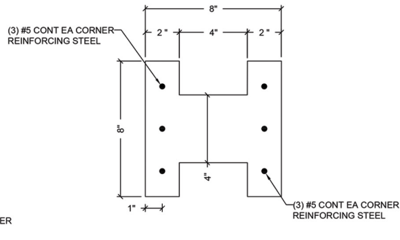
8 COLUMN SECTION 8x8 SCALE: 3"=1'-0"
