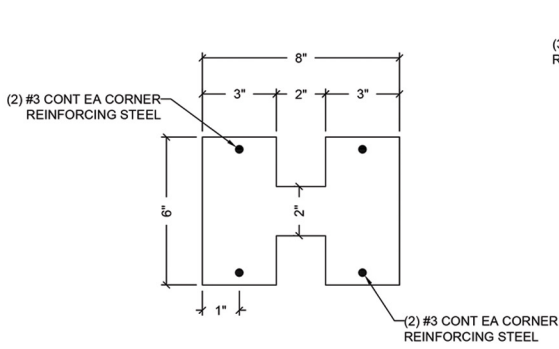
4 COLUMN SECTION 6x8 SCALE: 3"=1'-0"
