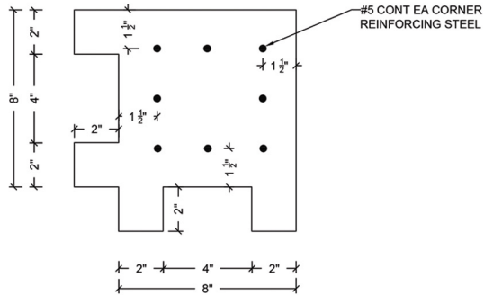
9 CORNER COLUMN SECTION 8x8 SCALE: 3"=1'-0"
